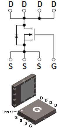
PDFN5×6-8L
