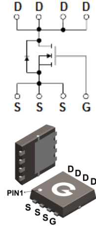
PDFN3×3-8L
