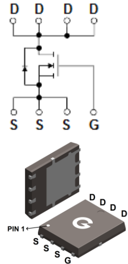
PDFN5×6-8L
