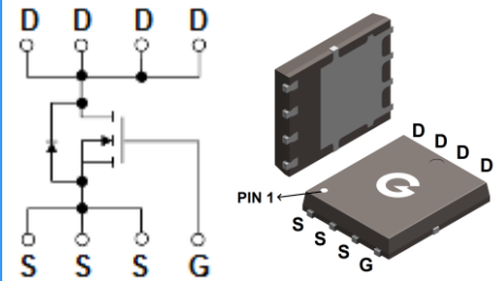
PDFN5×6-8L
