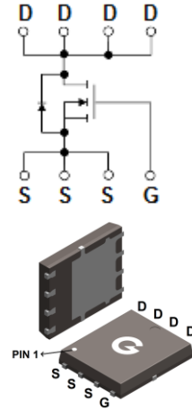
PDFN5×6-8L
