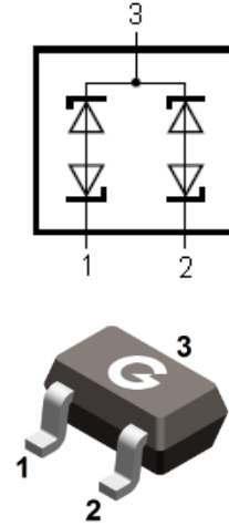
SOT-323
