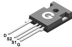
TO-247-4L
