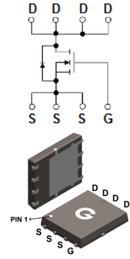
PDFN5×6-8L
