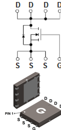
PDFN5×6-8L
