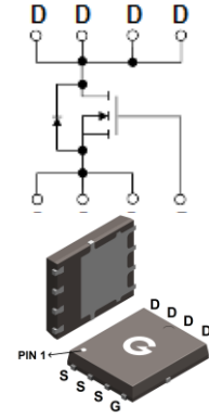
PDFN5×6-8L
