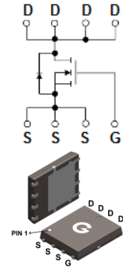
PDFN5×6-8L
